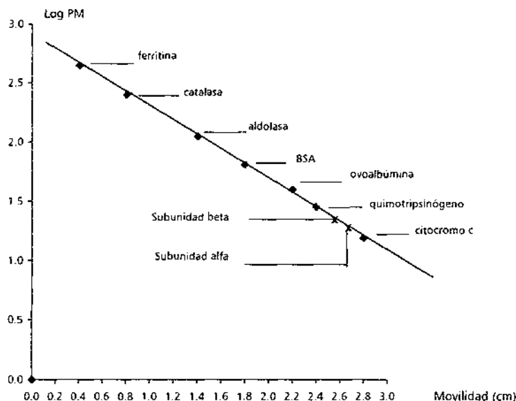
Fig. 9. Representación gráfica de la curva patrón, realizada para la estimación del peso molecular de las subunidades alfa y beta del hexámero de C-ficocianina, según la metodología de Ferguson modificada por Hames y Rickwood. 32
