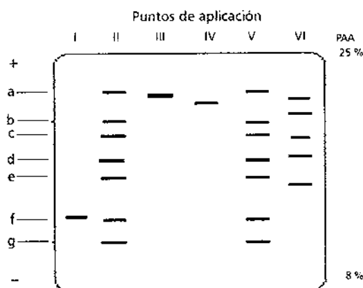
Fig. 5. Representación de la electroforesis nativa realizada a las fracciones F_1(\alpha\beta)_6 y agregado obtenidas por cromatografía de intercambio aniónico y a las fracciones \alpha y \beta obtenidas por filtración en gel. Se trabajó en sistema automatizado PhastSystem (Pharmacia) con Phastgel de un 8 a un 25 % de poliácridamida. Puntos de aplicación: I. Fracción F_1(\alpha\beta)_6 , II, V. Patrones (a: citocromo, b: quimotripsinógeno, c: ovoalbúmina, d: BSA, e: aldolasa, f: catalasa, g: ferritina). III. Fracción \alpha . IV. Fracción \beta . VI. Fracción agregado.
