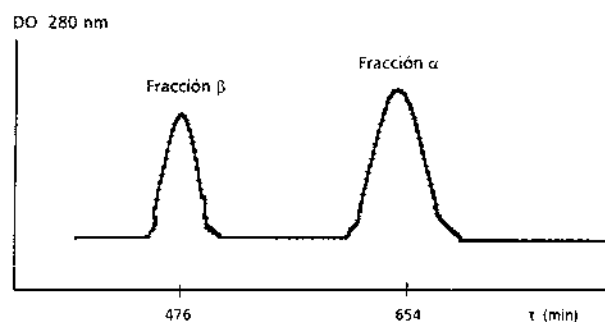
Fig. 7. Perfil de la cromatografía en filtración en gel. Se utilizó como gel Superdex-75 y una columna XK 26/100 con una altura de 90 cm. Se aplicaron 11 mL de muestra equilibrada a pH 3,6 y a un flujo de 0,55 mL/min.
