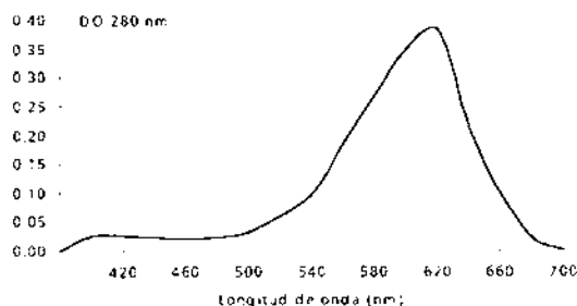
Fig. 3. Barrido de 400 a 700 nm de longitud de onda de la fracción F_1(\alpha\beta)_6 , obtenida por cromatografía de intercambio aniónico con gel DEAE Sepharosa FF, en una columna XK 26/20, con una altura de 10,0 cm.
