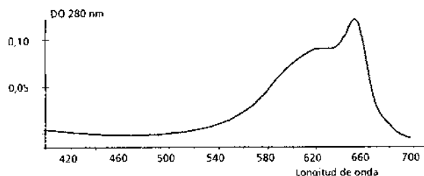
Fig. 4. Barrido de 400 a 700 nm de longitud de onda de la fracción agregado, obtenida por cromatografía de intercambio aniónico con gel DEAE Sepharosa FF, en una columna XK 26/20, con una altura de 10,0 cm.
