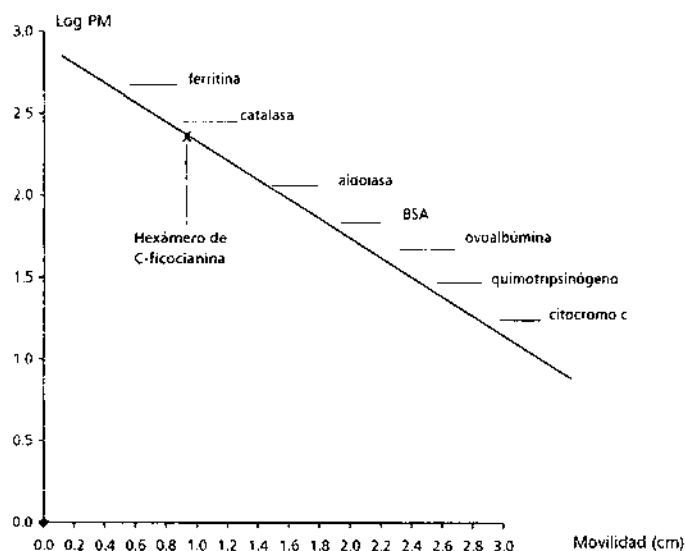
Fig. 8. Representación gráfica de la curva patrón, realizada para la estimación del peso molecular del hexámero de C-ficocianina, según la metodología de Ferguson modificada por Hames y Rickwood. 32
