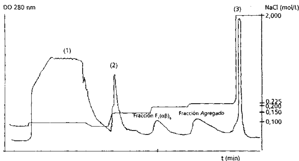
Fig. 2. Perfil de la cromatografía de intercambio aniónico con gel DEAE Sepharosa FF en una columna XK 26/20 con una altura de 10,0 cm. Se aplicaron 50 mL de muestra equilibrada a pH 7,2. La elusión se realizó con gradiente salino incrementado desde 0 hasta 2,0 mol/L, a un flujo de 5 mL/min.
