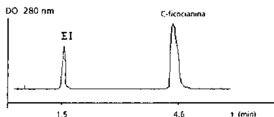
Fig. 6. Perfil de la Cromatografía Líquida de Alta Presión utilizando una columna de filtración en gel del tipo TSK-G3000SW de (4,6 x 300) mm, con una altura de 30 cm. Se aplicaron 50 \mu L de muestra equilibrada a pH 8,6 y a un flujo de 0,8 mL/min. El estándar interno correspondió a la proteína fibronectina con un peso molecular de 440 kDa.
