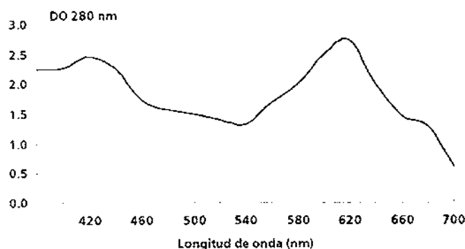
Fig. 1. Barrido de 400 a 700 nm de longitud de onda del crudo obtenido por el método de extracción de ficobiliproteínas por congelación-descongelación a -20 °C, para el proceso de purificación del hexámero de C-ficocianina.
